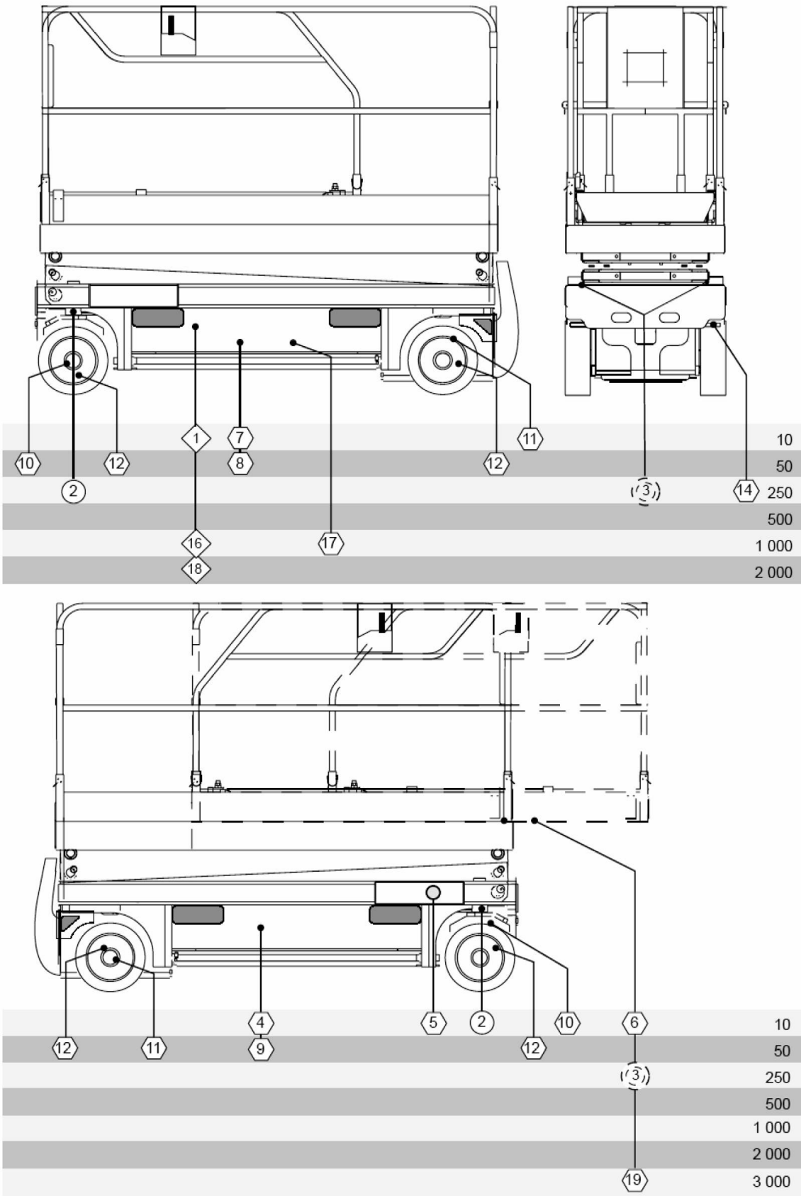
Рисунок 26. Схема технического обслуживания подъемника Compact 10N.
