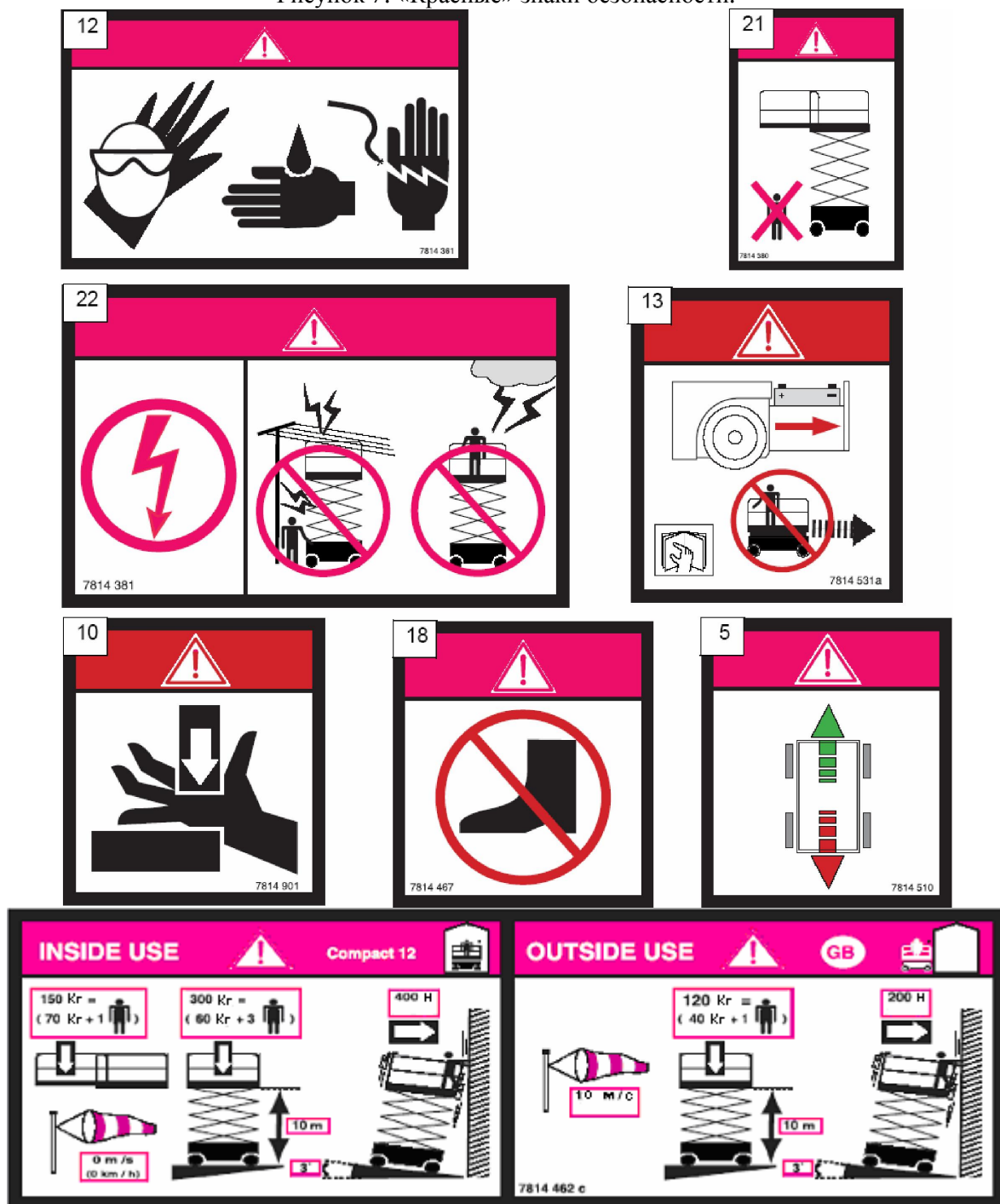
Рисунок 7. «Красные» знаки безопасности.
