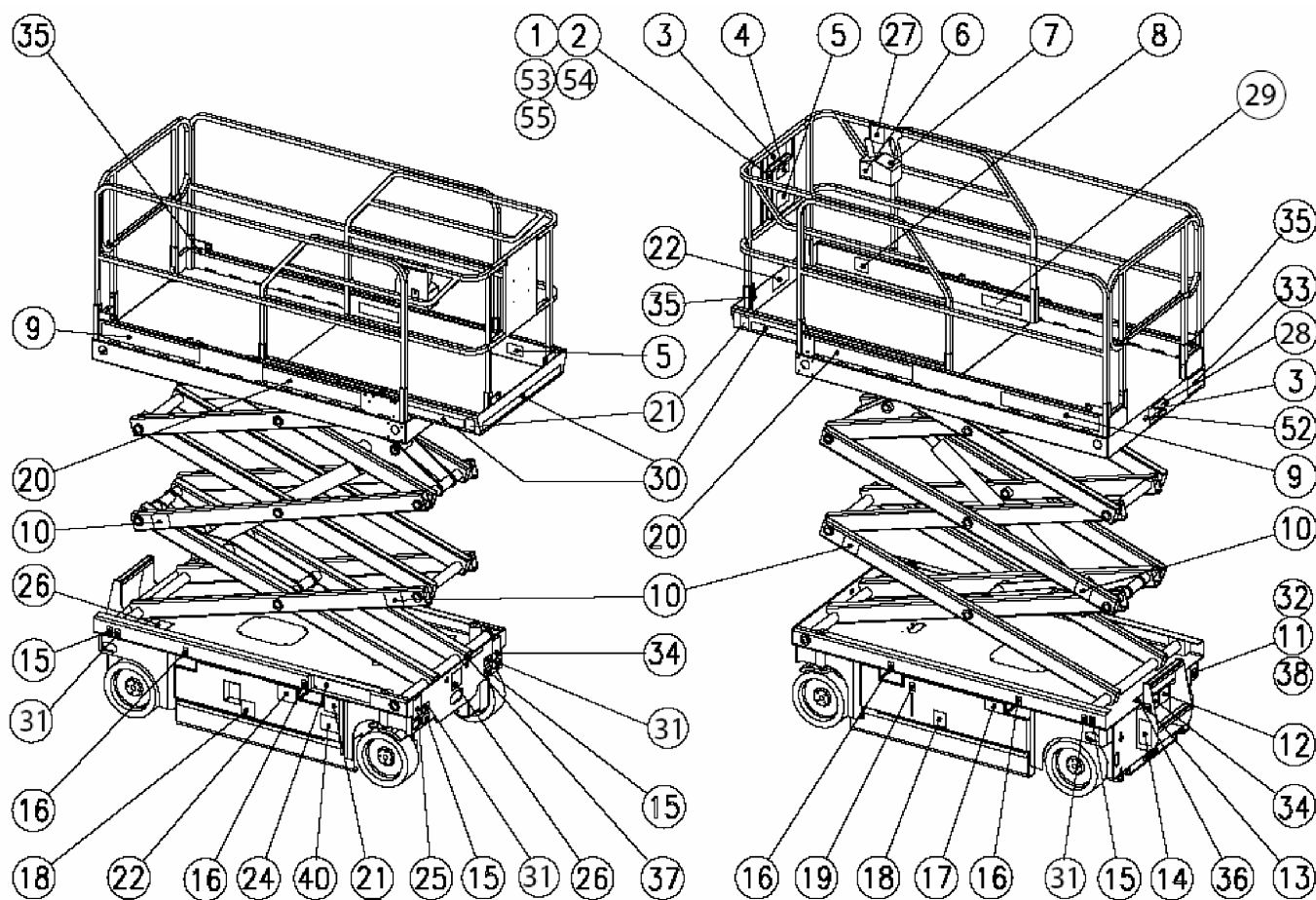
Рисунок 8. Расположение знаков безопасности.
