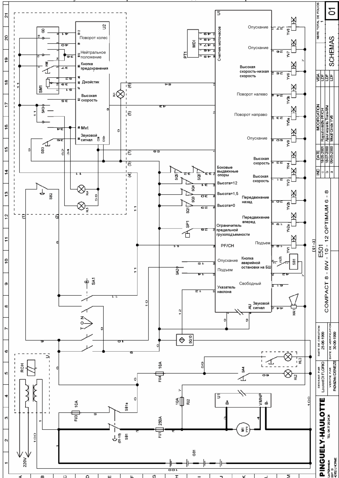
Рисунок 31. Электрическая схема подъемника Compastr 10N.
